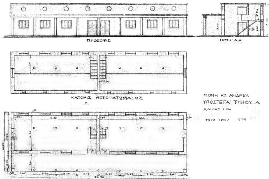
Σχ. 16. Σχέδιο υποστέγων (δωματίων φιλοξενίας) τύπου Α, του 1946. Αφοι Μιχαηλίδη, κατόψεις, τομή και όψη. Το κτήριο δεν κατασκευάστηκε (Αρχείο Μονής Απ. Ανδρέα).
