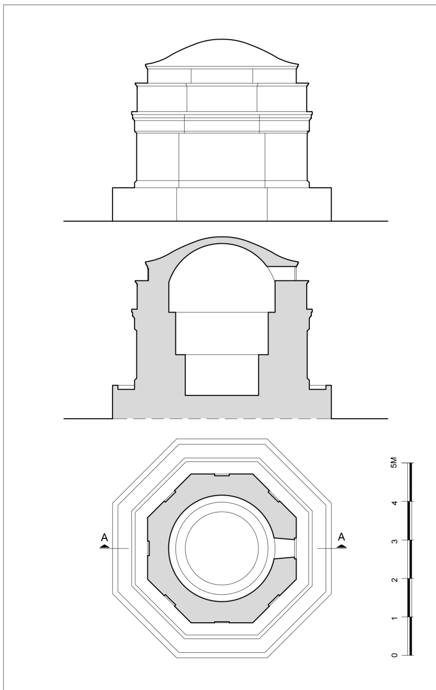
Σχ. 12. Κρήνη αυλής, κάτοψη-τομή-όψη (Μελέτη Πανεπιστημίου Πατρών).
