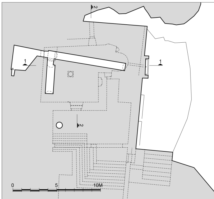
Σχ. 3. Μεσαιωνικός ναός, κατόψεις (Μελέτη Πανεπιστημίου Πατρών).
