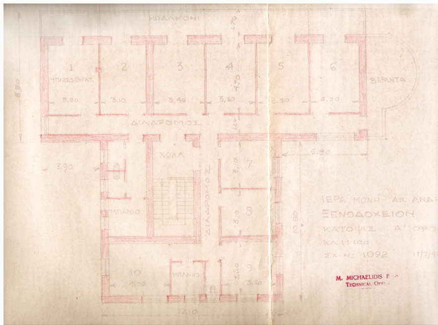
Σχ. 19. Σχέδιο ξενοδοχείου του 1946. Αφοι Μιχαηλίδη (M. Michaelides Bros Technical Office), κάτοψη Α' ορόφου. Το κτήριο δεν κατασκευάστηκε (Αρχείο Μονής Απ. Ανδρέα).
