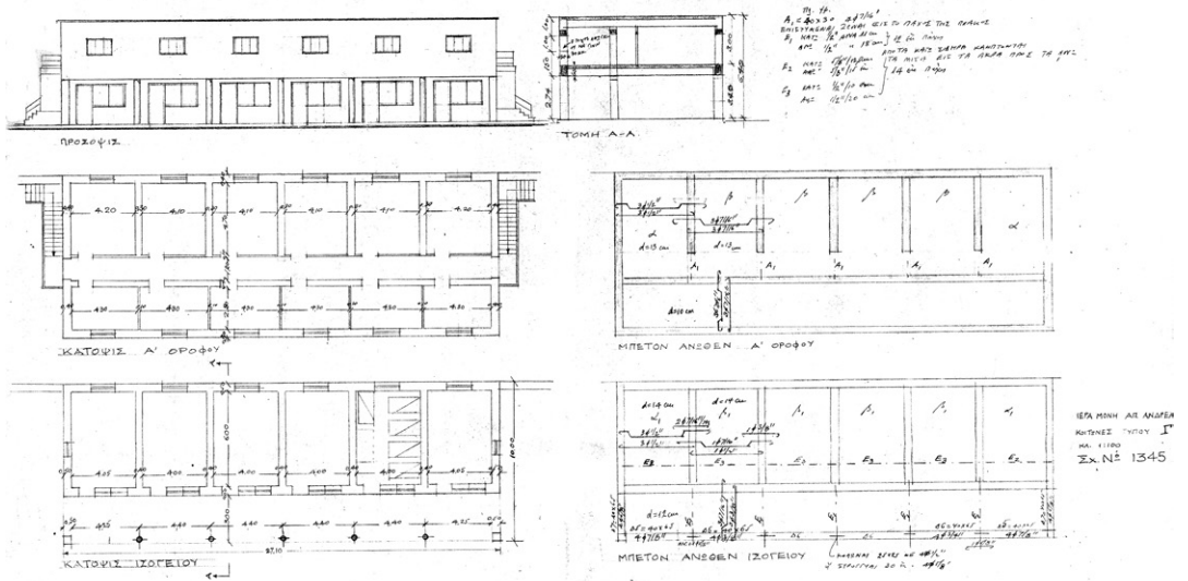
Σχ. 18. Σχέδιο υποστέγων (δωματίων φιλοξενίας) τύπου Γ, του 1946. Αφοι Μιχαηλίδη, κατόψεις, τομή, ύψη και στατικά σχέδια. Το κτήριο δεν κατασκευάστηκε (Αρχείο Μονής).
