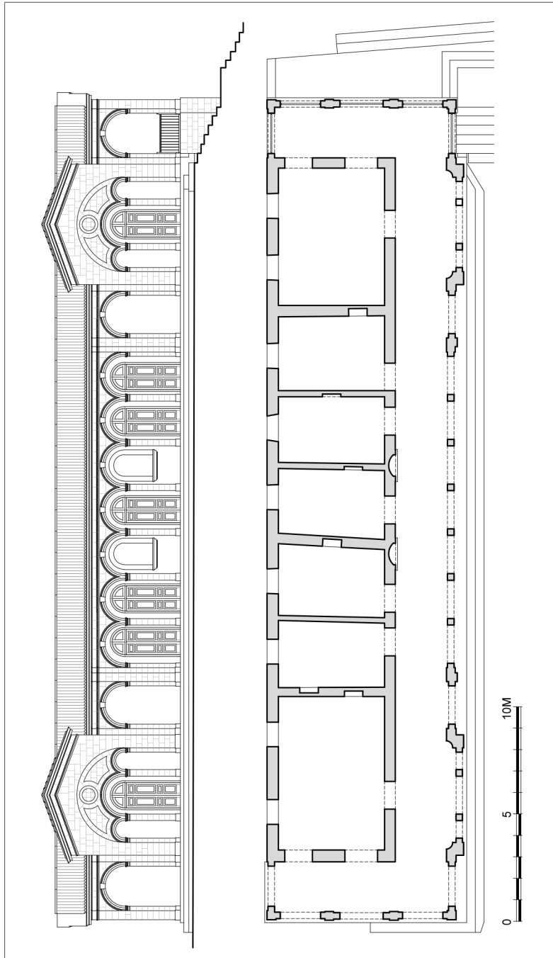
Σχ. 11. Κτήριο δωματίων φιλοξενίας και Συνοδικού του 1919, αρχιτέκτων Θ. Φωτιάδης, κά- τοψη και νότια όψη (Μελέτη Πανεπιστημίου Πατρών).
