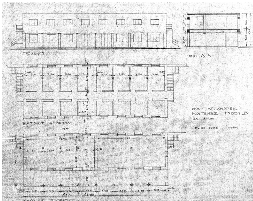
Σχ. 17. Σχέδιο υποστέγων (δωματίων φιλοξενίας) τύπου Β, του 1946. Αφοι Μιχαηλίδη, κατόψεις, τομή και όψη. Το κτήριο δεν κατασκευάστηκε (Αρχείο Μονής Απ. Ανδρέα).
